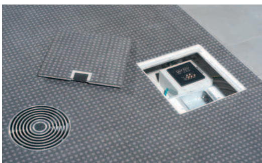
Verbund-Doppelboden in Konferenzraum belegt mit dessiniertem Teppichbelag mit eingebauter Serviceöffnung und Lüftungsauslass
