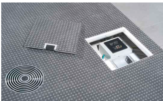
Verbund-Doppelboden in Konferenzraum belegt mit dessiniertem Teppichbelag mit eingebauter Serviceöffnung und Lüftungsauslass
